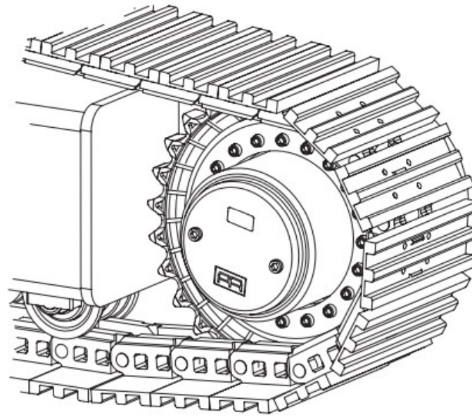
Piñón para cadena de arrastre
